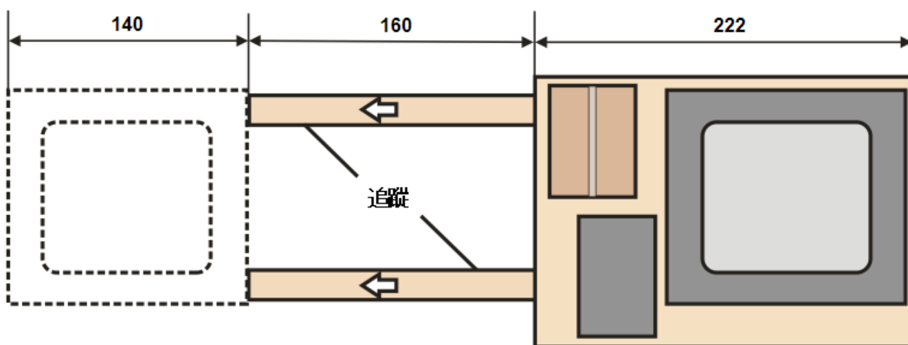
圖4 卸貨尺寸—頂視圖
