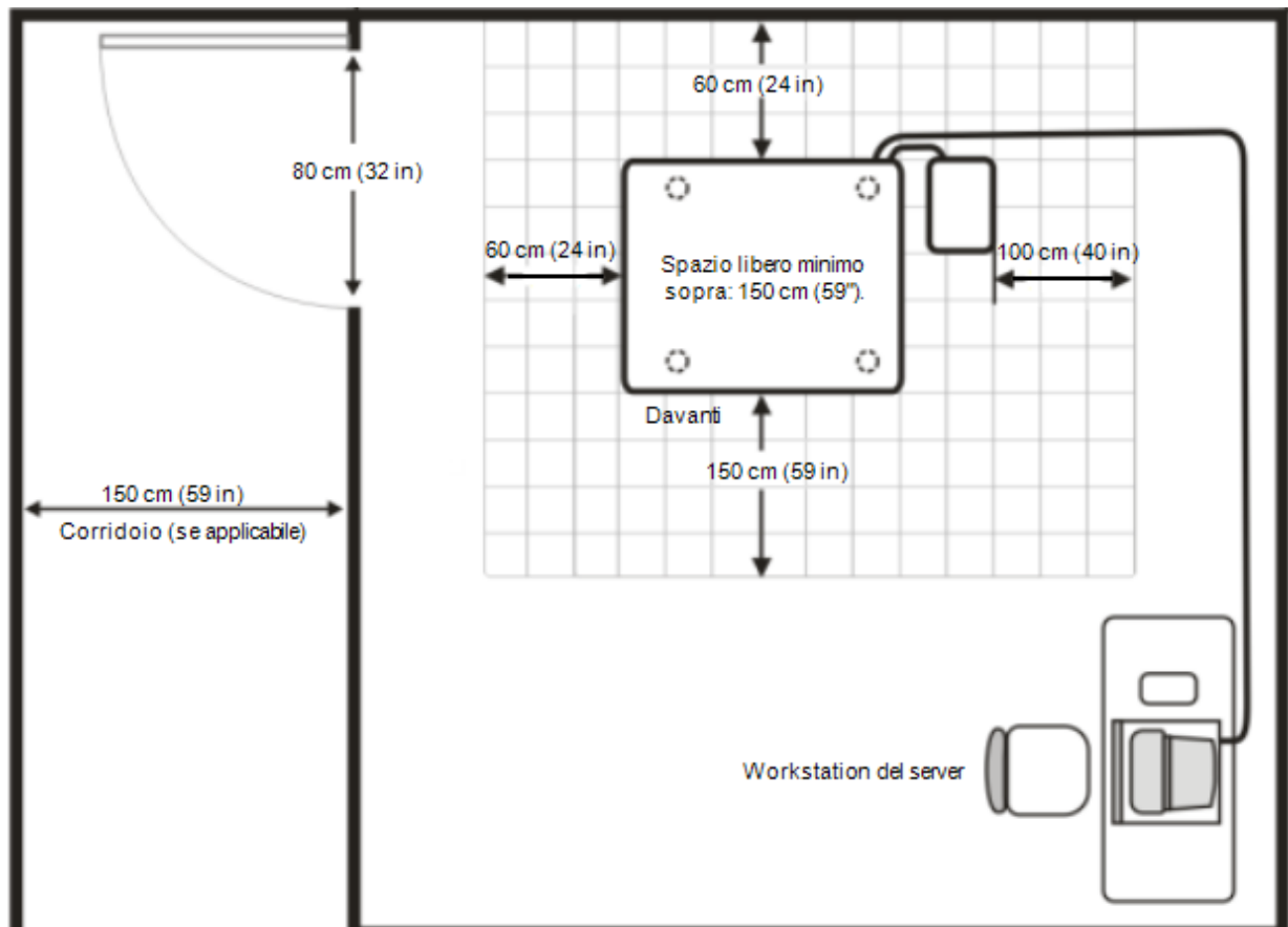
Figura 3 Esempio di planimetria della stampante (non in scala)
