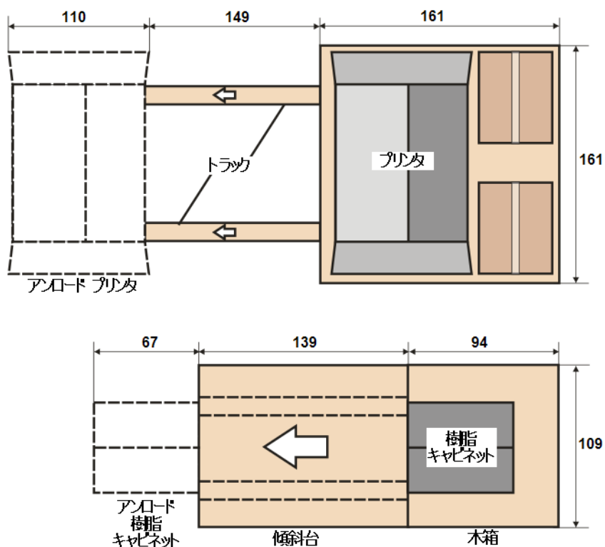
図 2 荷降ろし寸法—上方より見た図
