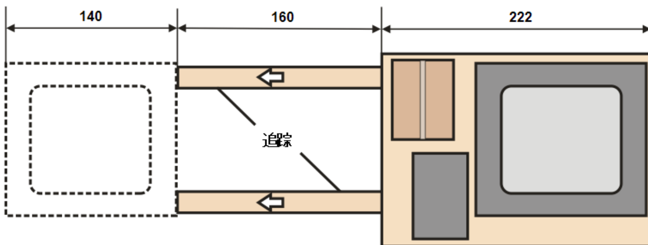
图4 卸货尺寸—顶视图
