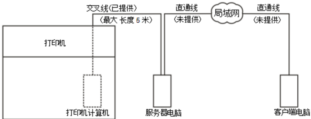
图9 网络安装
