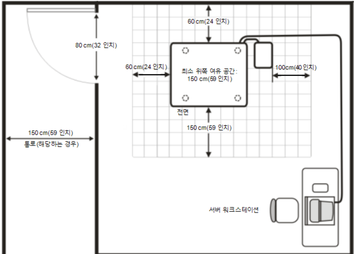
그림 3 프린터 평면도(샘플, 비례가 아님)
