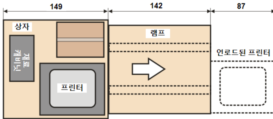
그림 2 언로드 치수 -상단 보기
