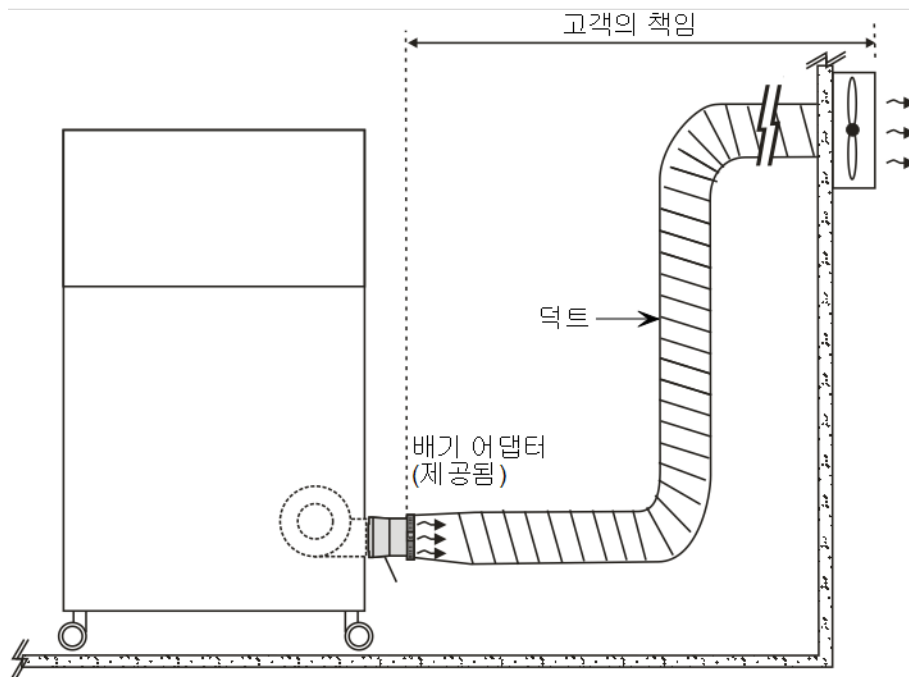
그림 6 프린터 배기 시스템
