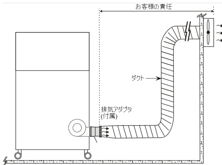
図 5 プリンタの排気システム
